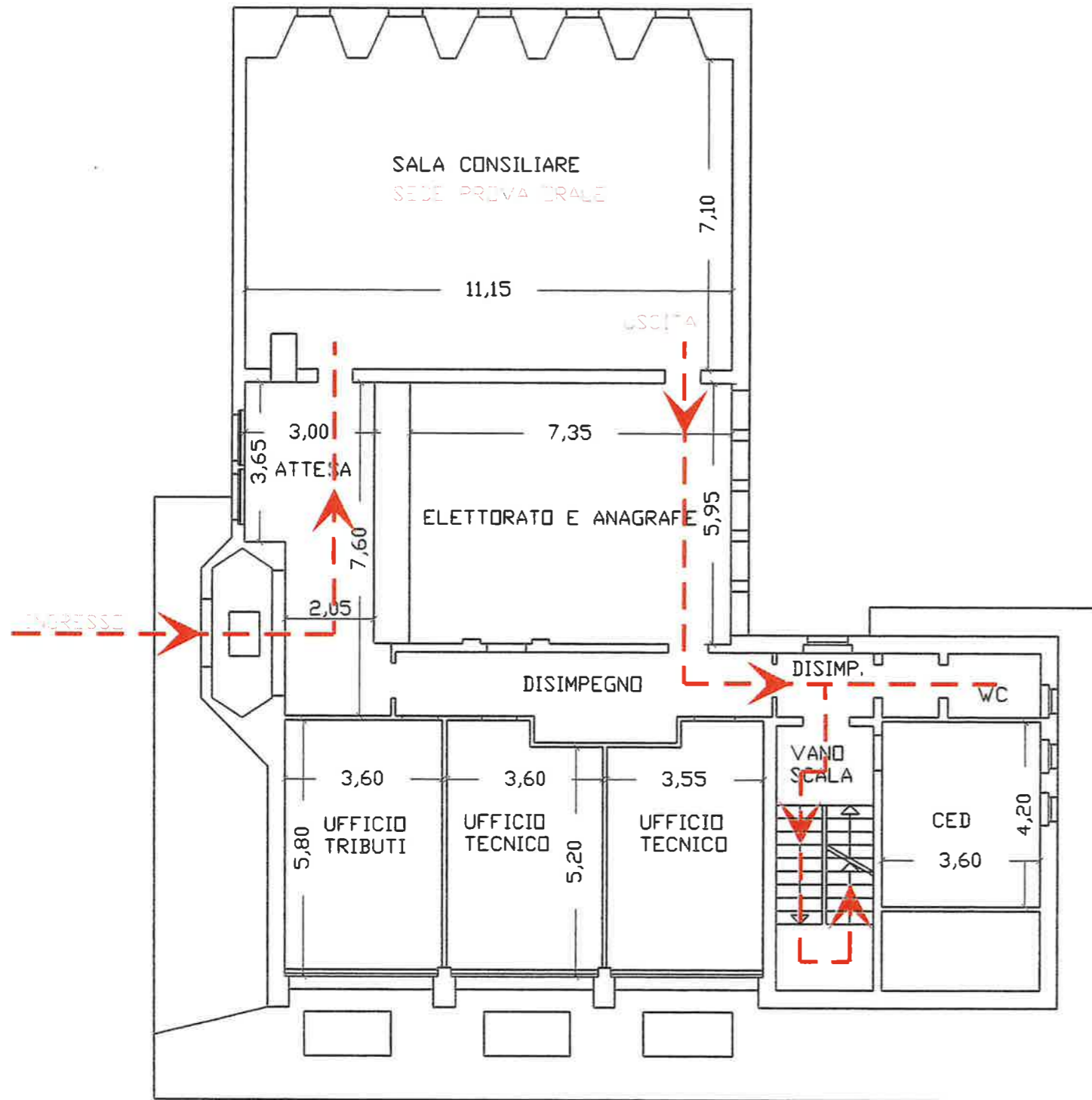
PIANO RIALZATO STATO DI FATTO
