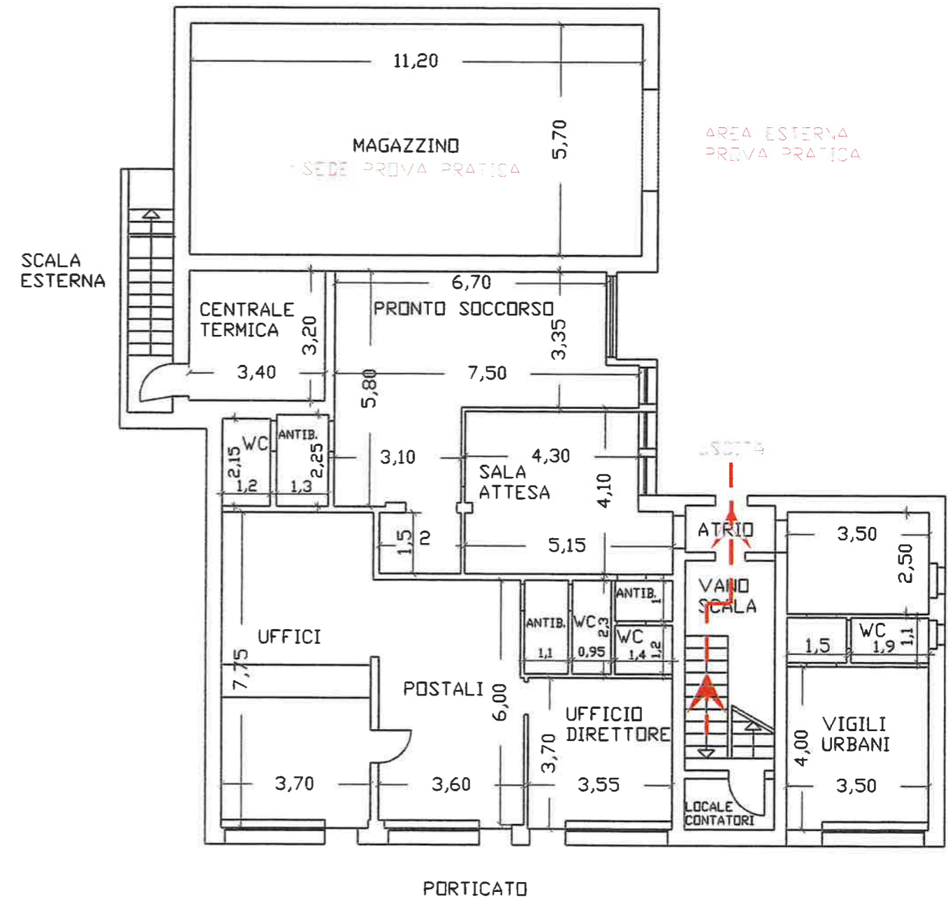
PIANO TERRA STATO DI FATTO
